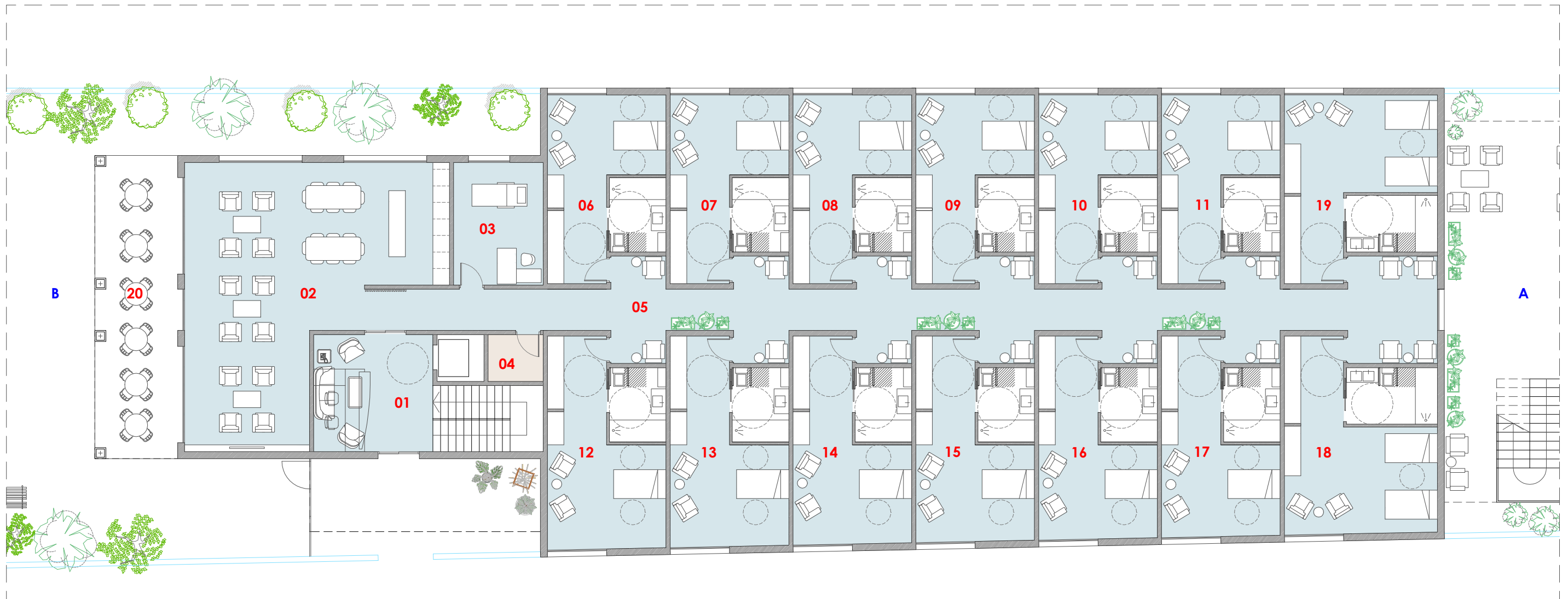
PLANTA GENERAL UNIDAD DE CONVIVENCIA
